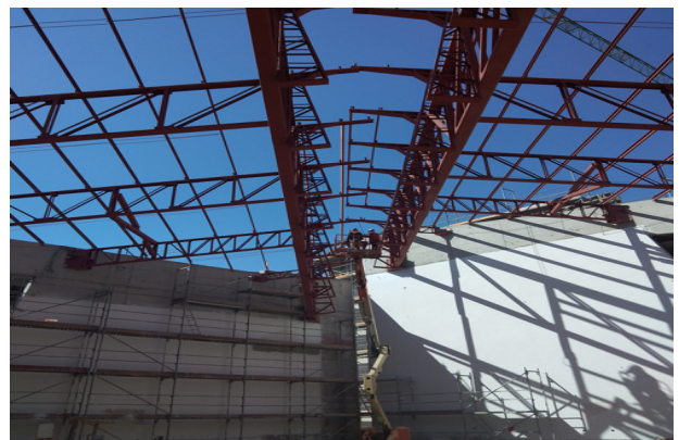
Montaje de costaneras, eje central, templo mayor.
